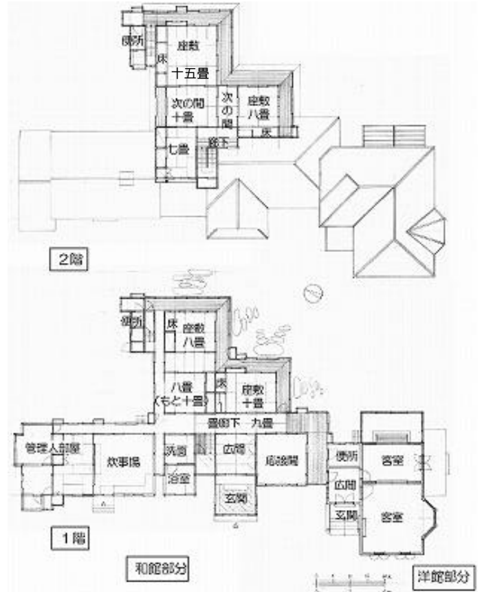
図2 豊門会館本館 平面図
