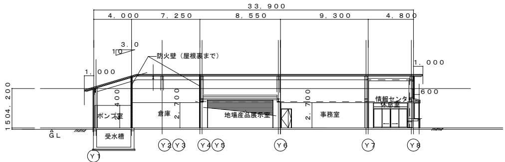
断面図 1:200
