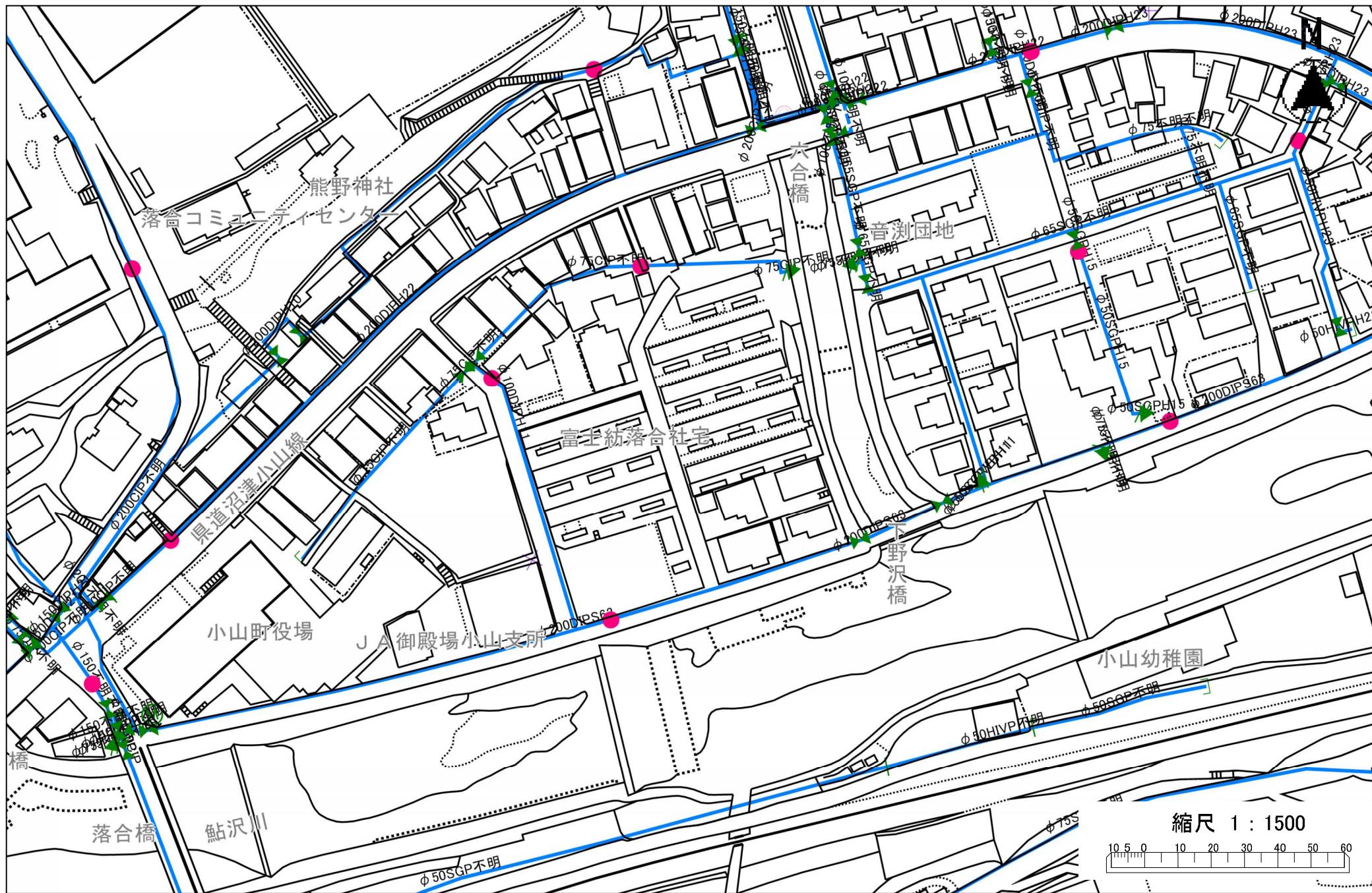
上水道配管図
