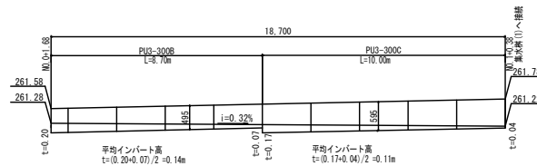
PU3-300B_300C展開図 H=1:100 V=1:50
