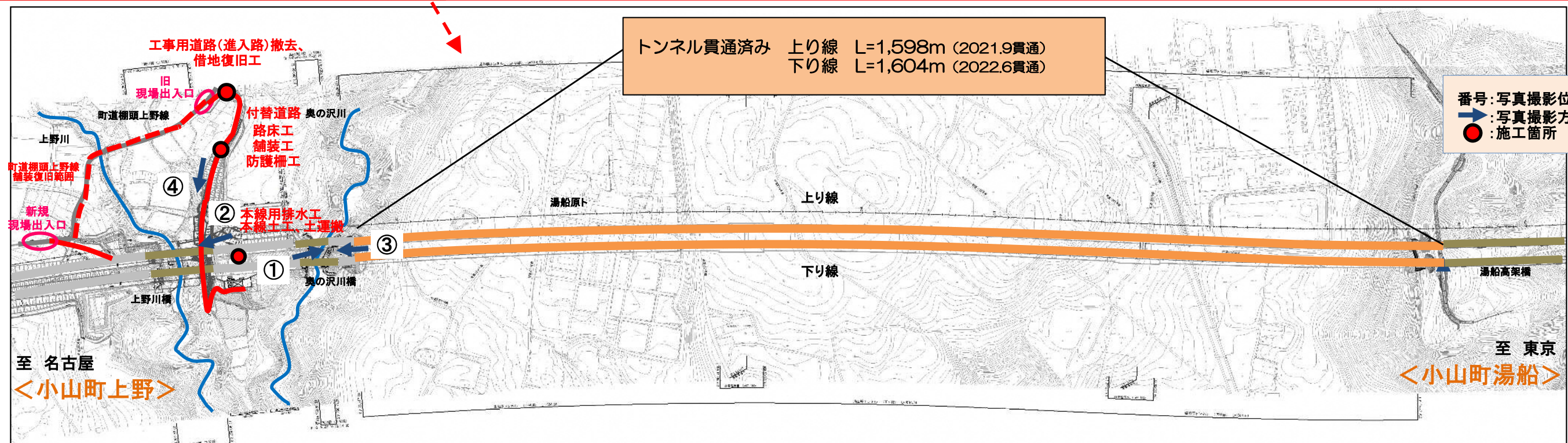
①西側トンネル坑口
