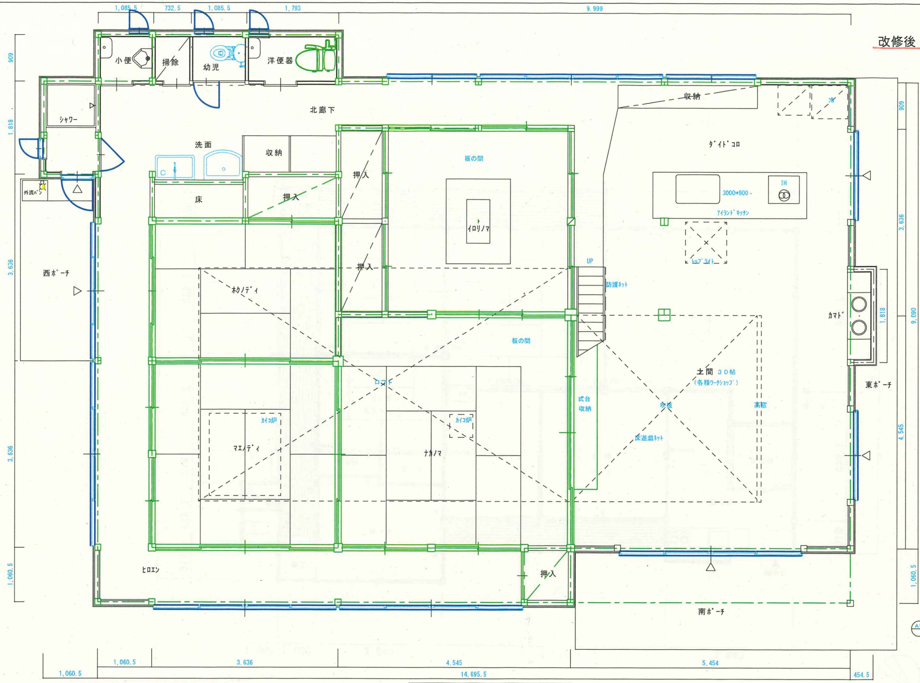
1階平面図 S = 1/50
